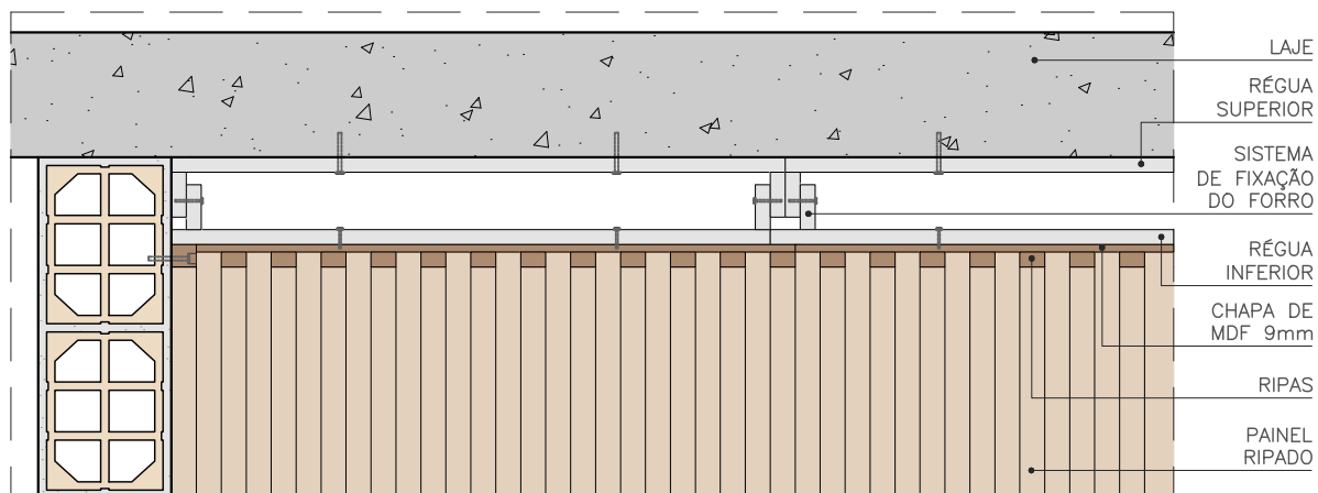
VISTA ESC. 1:10
