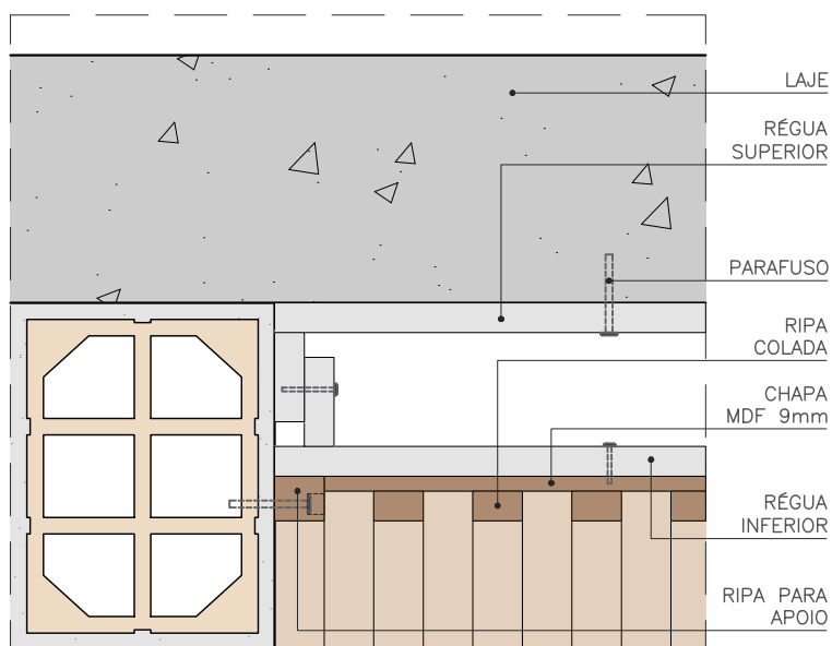
DET. FIXAÇÃO DO FORRO ESC. 1:5
