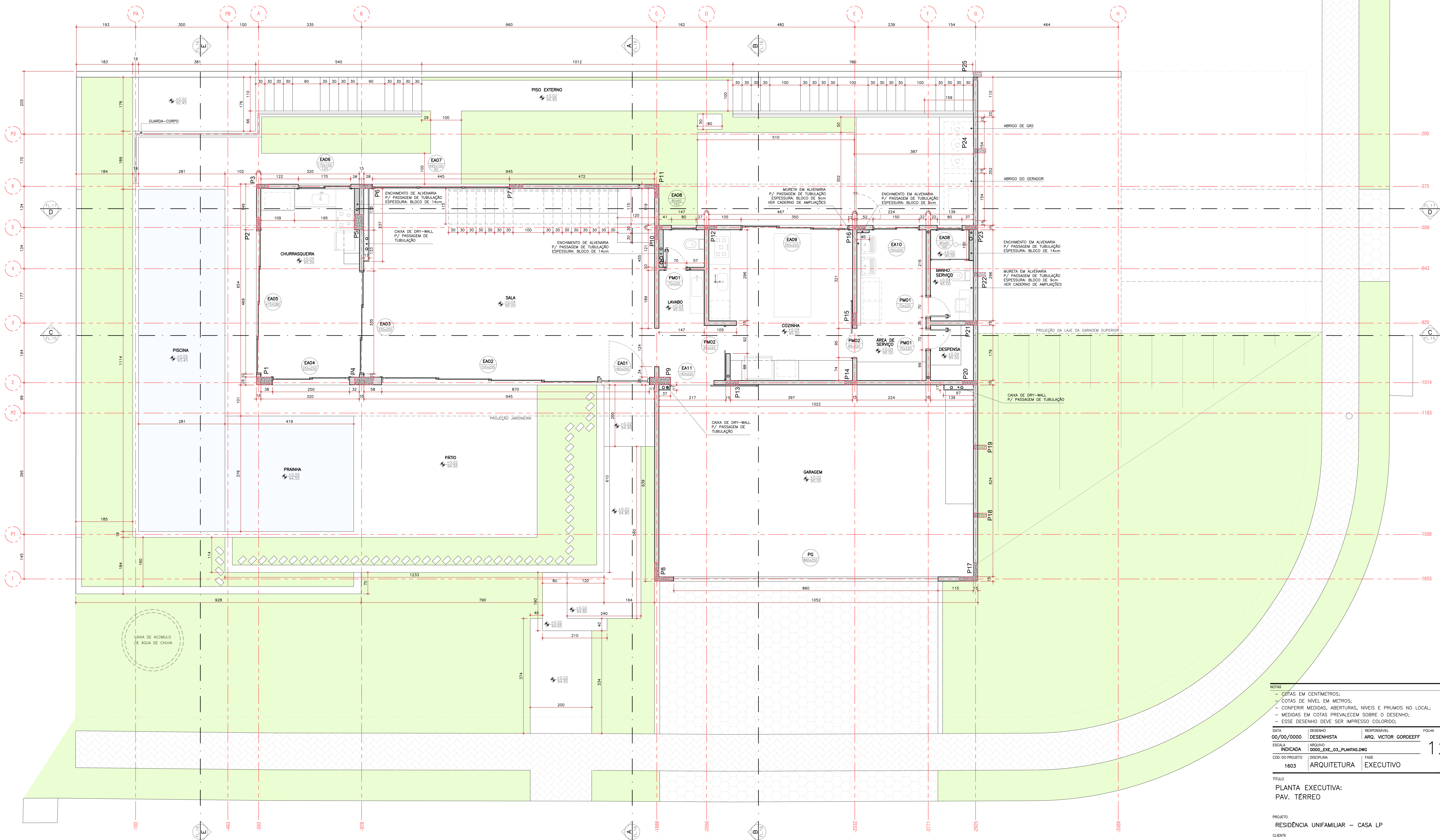
PLANTA EXECUTIVA – PAV. TERREO 1:50
